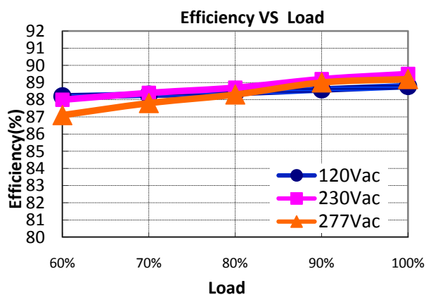
X6-060Y050( I_o=1.20A )
