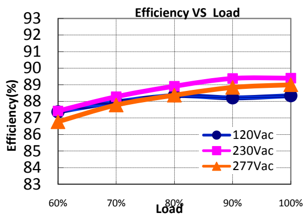
X6-060Y050( I_o=1.20A )
